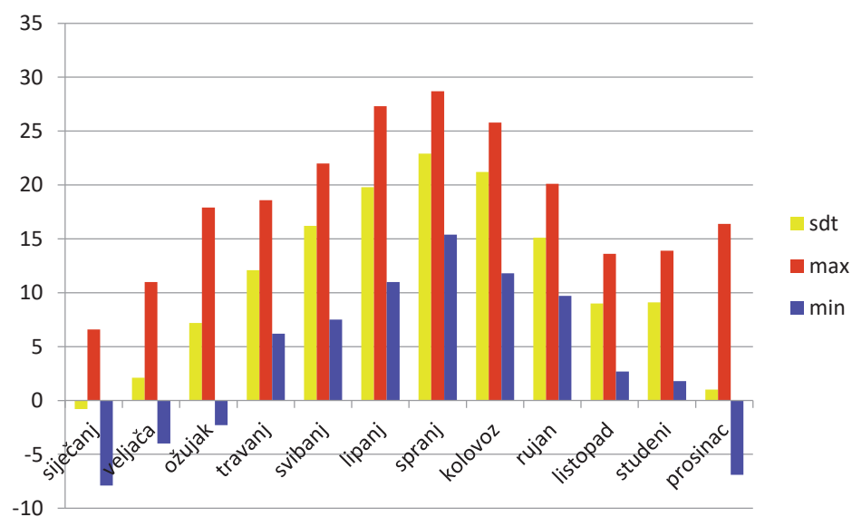
Slika 6. Temperature u 2011. godini – mjerna postaja Našice
